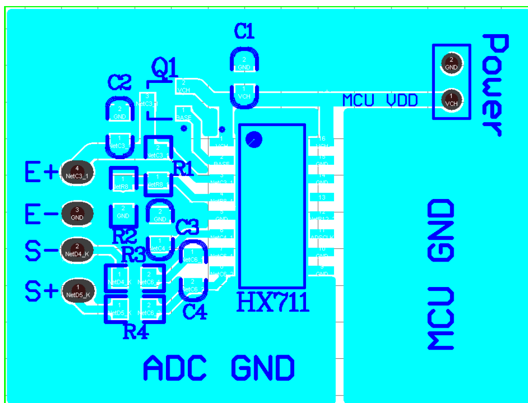
图五 与 HX711 相关部分的单层 PCB 板参考设计板图
