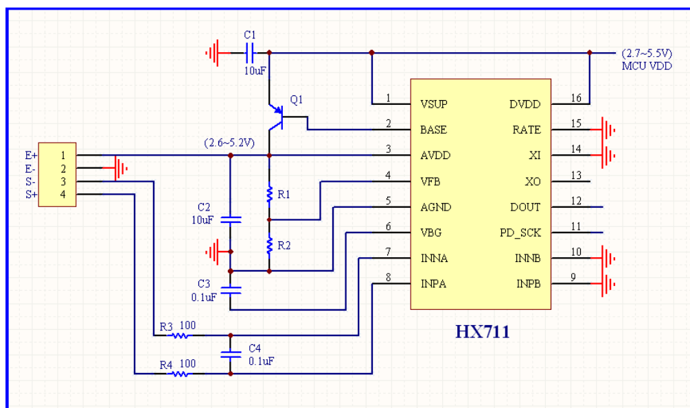
图四 与 HX711 相关部分的 PCB 板参考设计线路图
