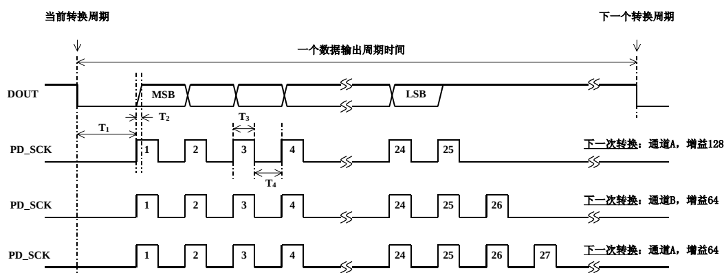
图二 数据输出，输入通道和增益选择时序图
