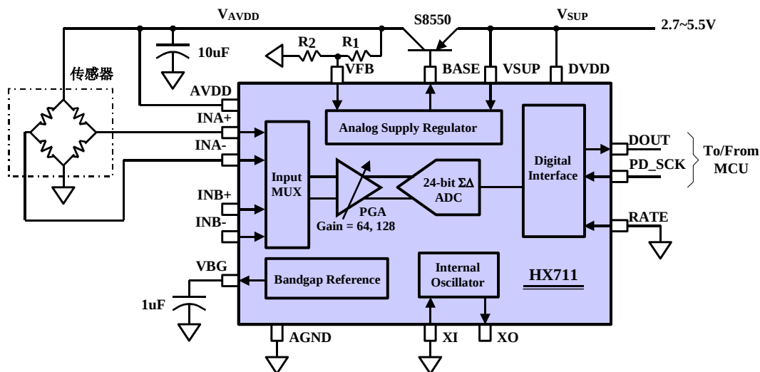
图一 电子秤应用典型方案图
